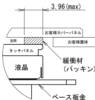
【お客様カバーパネル付き筐体の構造例】
