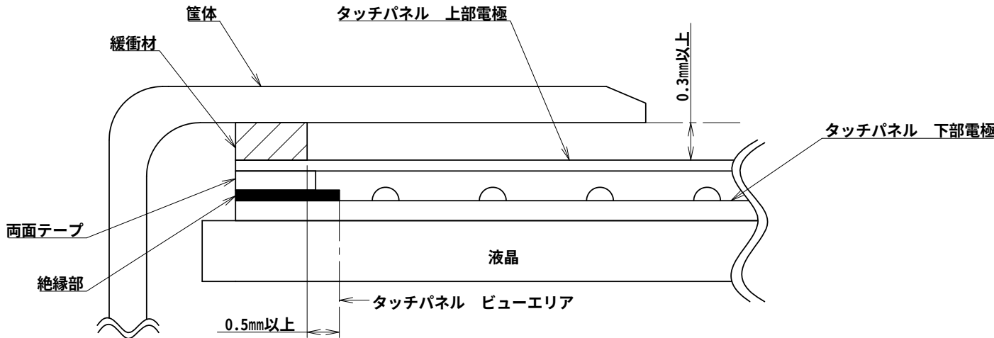
筐体設計参考図
