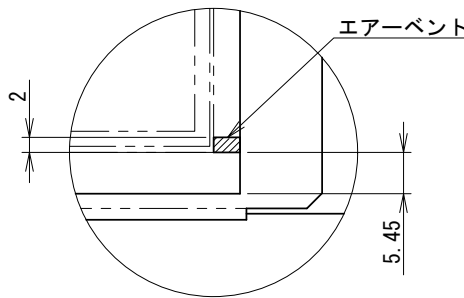
詳細図 A スケール 1 : 1
